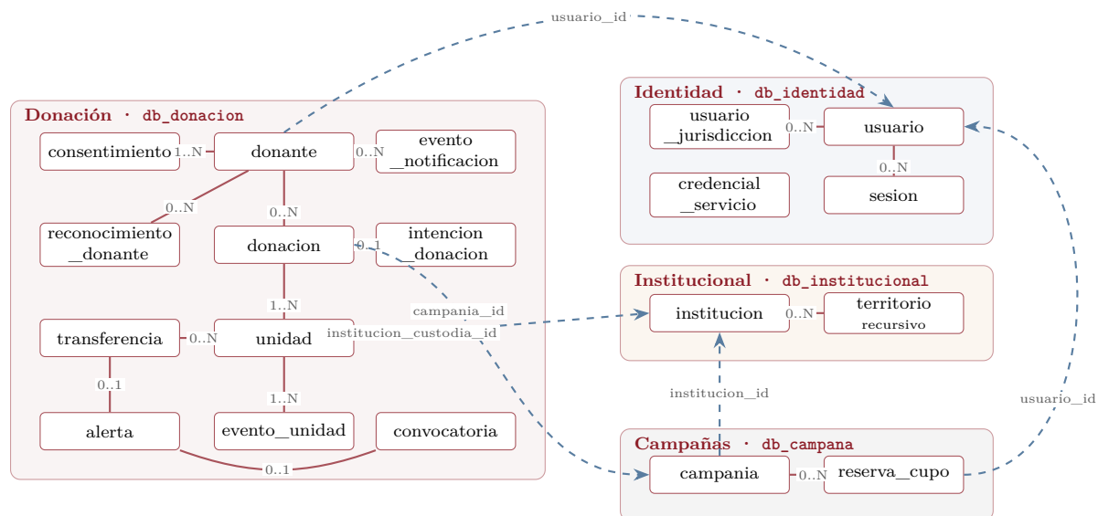
Figura 1: Modelo conceptual. Las líneas continuas son relaciones internas con integridad referencial garantizada por el motor. Las discontinuas son referencias que cruzan la frontera: se almacenan como identificador y se resuelven por contrato, sin clave foránea, porque las bases son independientes. La figura muestra las cinco más significativas y omite la relación recursiva de territorio consigo mismo; el diccionario de datos declara todas. Las referencias territoriales no se dibujan porque viajan como ruta DIVIPOLA y no como identificador. Se omiten los catálogos, las cuatro series de la bitácora, operacion_idempotente y umbral_inventario , que no participan de relaciones que expliquen el dominio.
